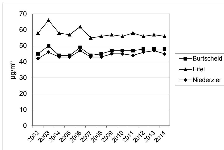
Abbildung 50: Ozon in der Außenluft in µg/m 3 , Jahresmittelwerte, Messstationen: Niederzier, Eifel (Simmerath) und Aachen-Burtscheid, 2002 – 2014
